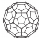
fullerene
